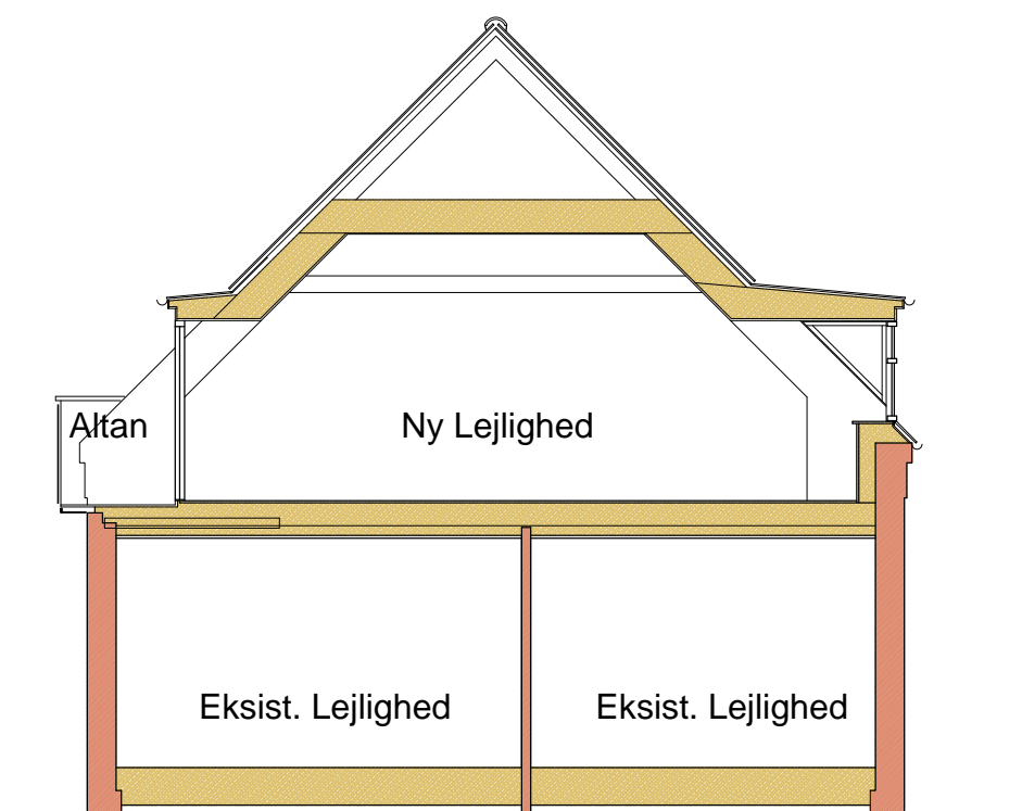
Snit Mål 1 : 100
