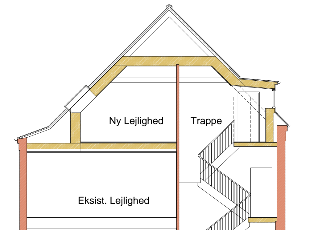
Snit Mål 1 : 100
