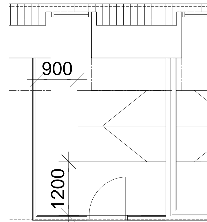
Plan udsnit
