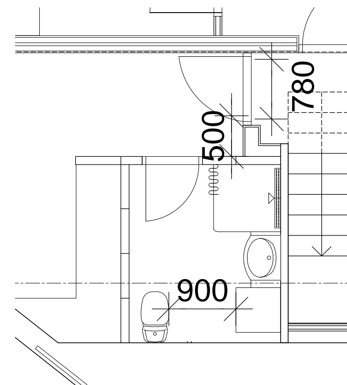
Plan udsnit
