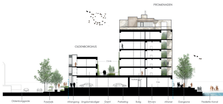
Principsnit af bebyggelsen "Promenaden" og "Oldenborghus". Den eksisterende by ligger til venstre.
