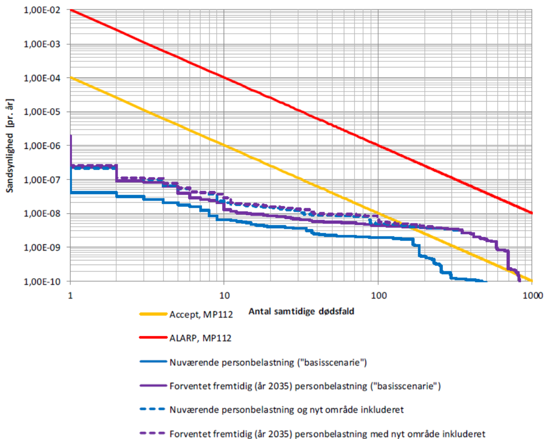
Figur 2.1 Den samfundsmæssige risiko baseret på de eksisterende aktiviteter omkring Fredericia Rangerbanegård med og uden etablering af et nyt standsningsområde for persontog tæt ved henstillingsområdet for farligt gods (blå kurver) og tilsvarende ved fremskrivning til et øget befolkningsgrundlag i år 2035 (lilla kurver).
