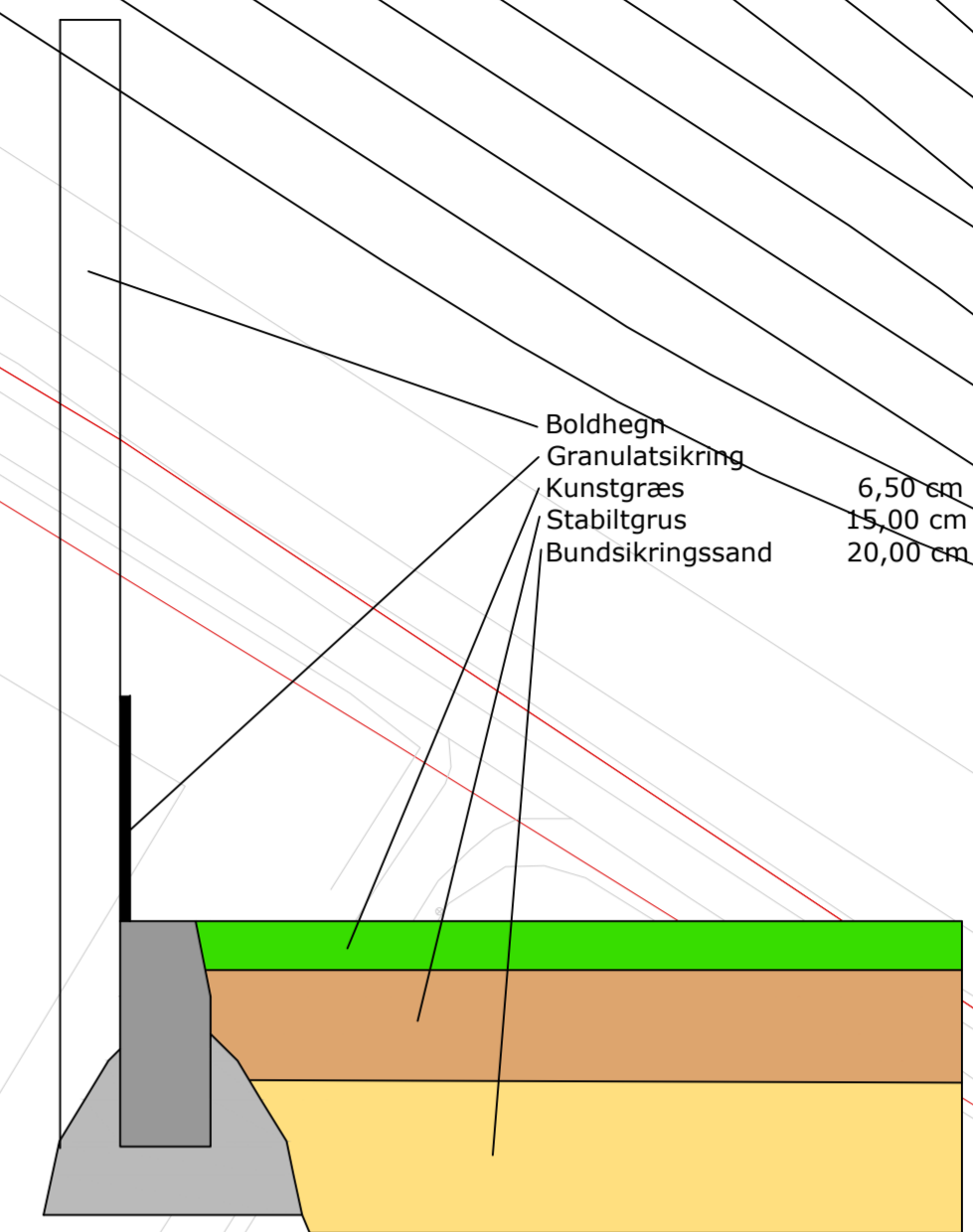
Principskitse 1:10
