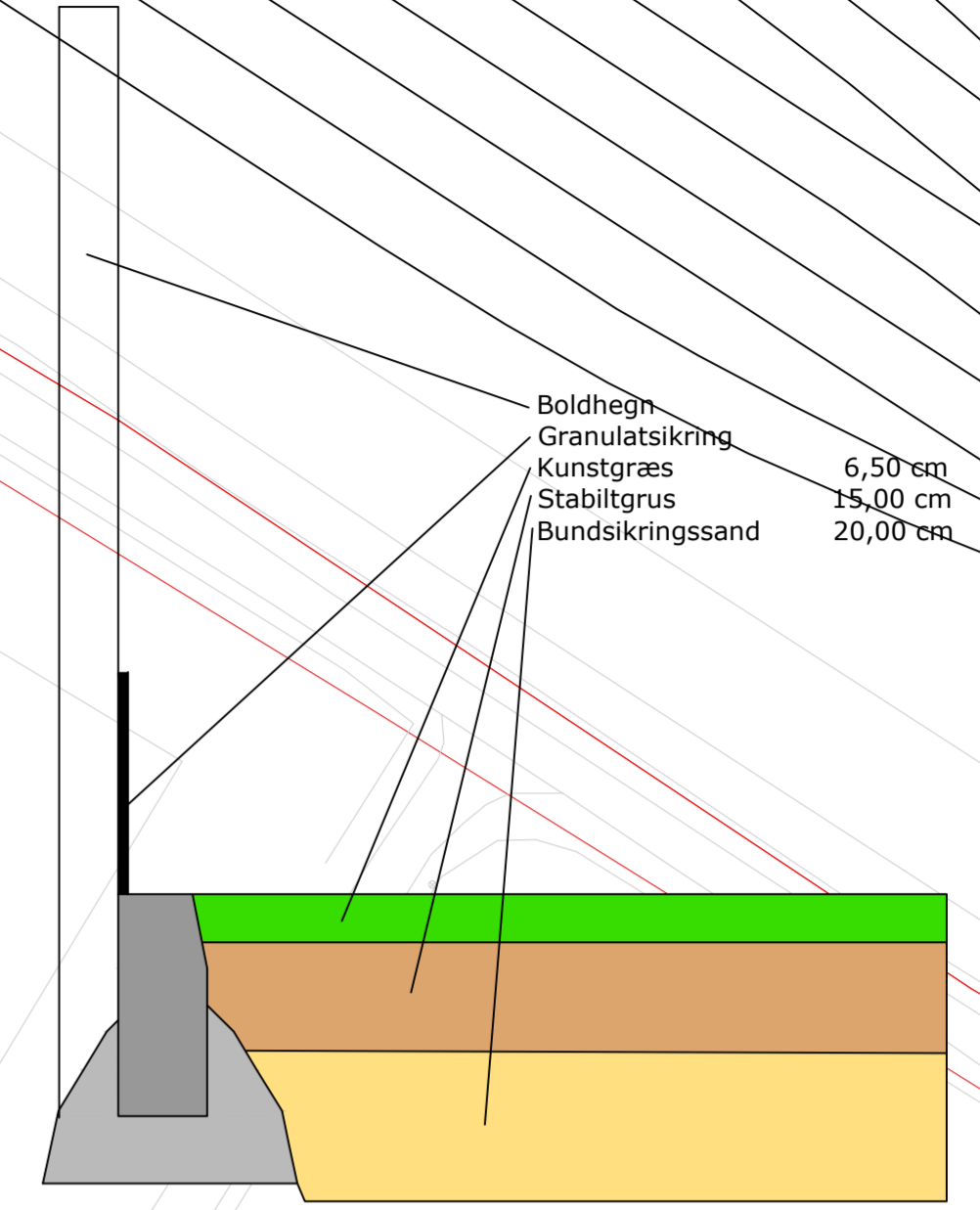
Principskitse 1:10
