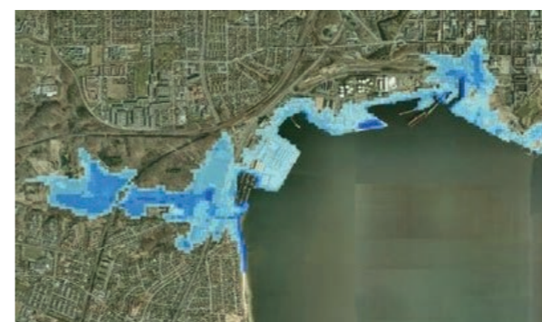
FIGUR 6 SAMMENLIGNING AF EN EKSTREM STORMFLOD - NUTID (2012 VS 2019)
