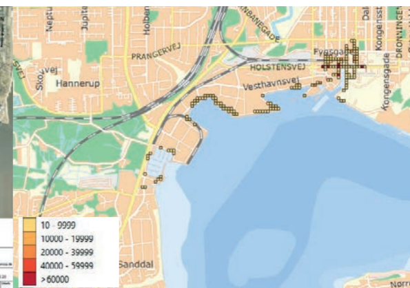
FIGUR 13 SAMMENLIGNING AF RISIKOKORT VED EN 100-ÅRS STORMFLOD - NUTID (2015/2019)
