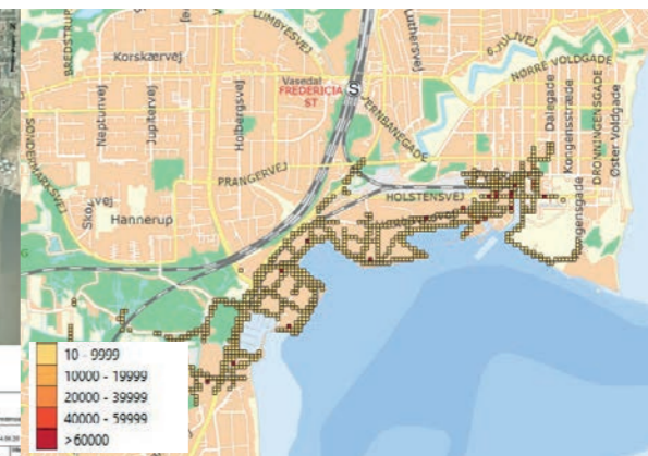
FIGUR 15 SAMMENLIGNING AF RISIKOKORT VED EN 100-ÅRS STORMFLOD - 2100 VS 2115 (2012-DATA VS 2019-DATA)
