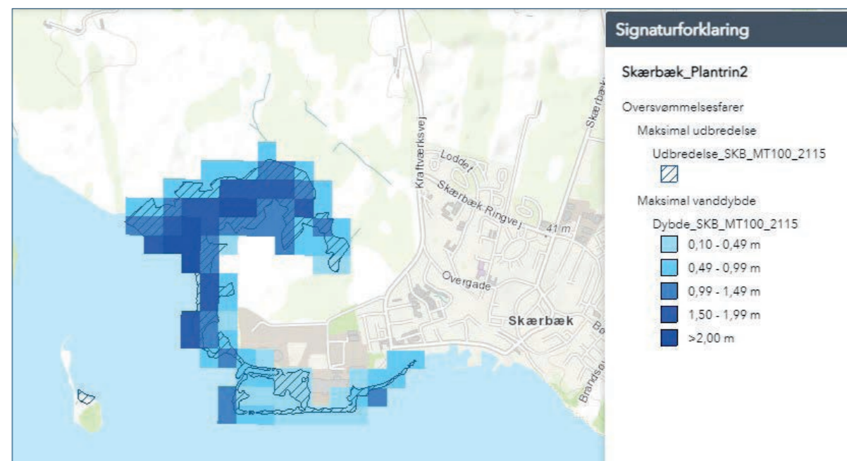
FIGUR 11 SKÆRBÆK 100-ÅRS STORMFLOD 2015 (2019-DATA)
