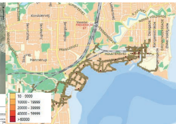
FIGUR 14 SAMMENLIGNING AF RISIKOKORT VED EKSTREM STORMFLOD - NUTID (2012-DATA VS 2019-DATA)
