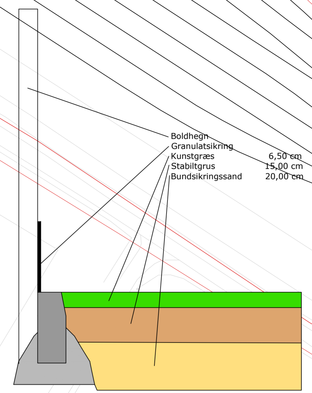
Principskitse 1:10
