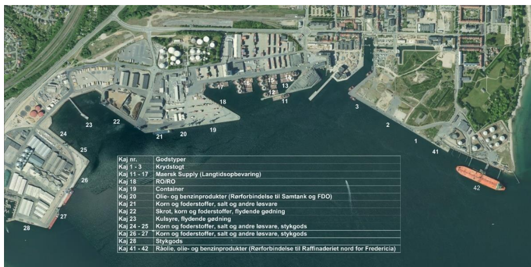
Figur 1-1: Eksisterende forhold med kaj nummerering.
