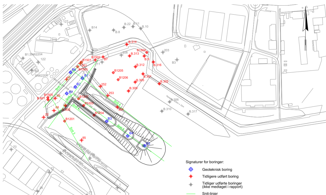
Figur 4-4: Placering af geotekniske boringer (Ref. /6/).
