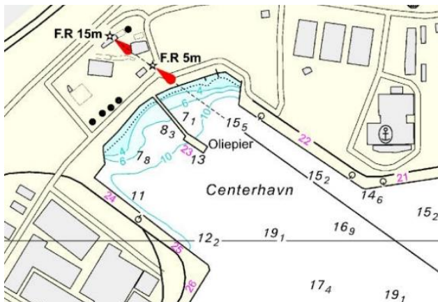
Figur 4-19: Vise vanddybderne ved Centerhavnen (Ref. /7/).
